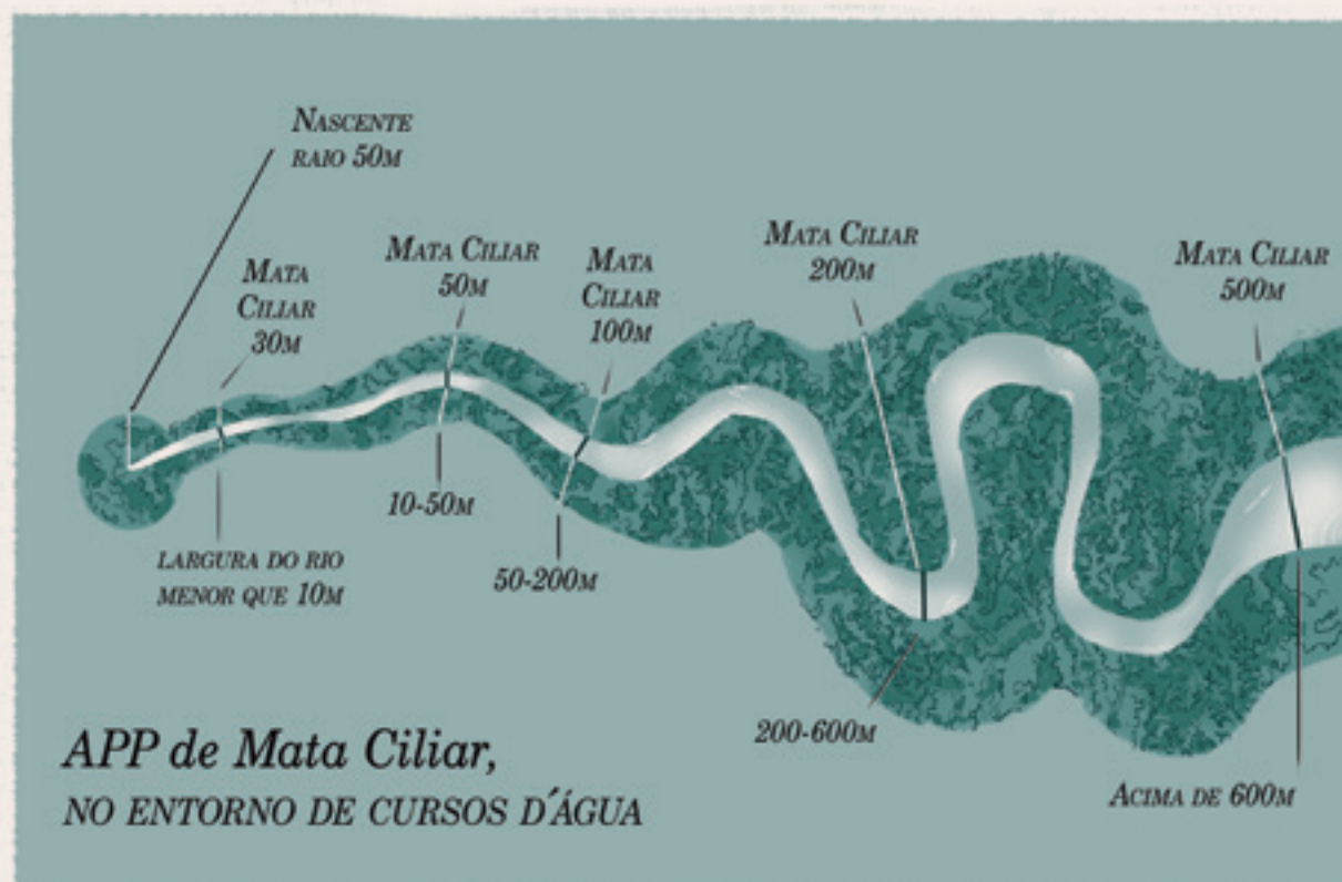
Figura 16 – Métricas de largura da faixa de APP de acordo com a largura do curso d'água. As faixas de proteção devem ser medidas a partir da borda da calha do leito regular do rio, onde corre água durante o período da seca.
